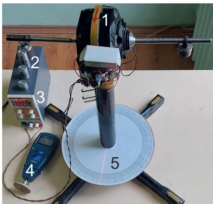
Рис.3. Фото установки.
