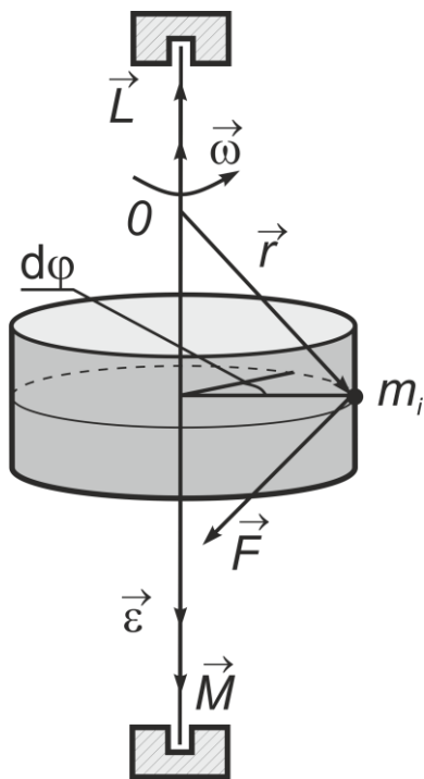
Рис. 1. Кинематические ( d\varphi , \omega , \varepsilon ) и динамические ( F , M , L ) характеристики вращательного движения твердого тела
