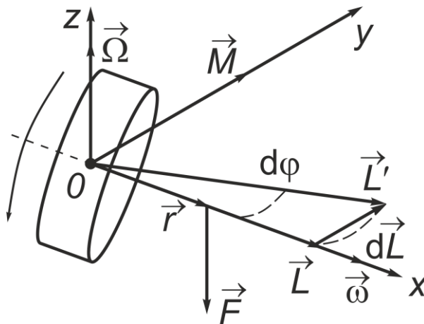
Рис.2. Прецессия гироскопа под действием силы F .
