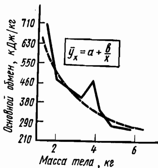
Рис. 32. Зависимость величины основного обмена обезьян от массы их тела
