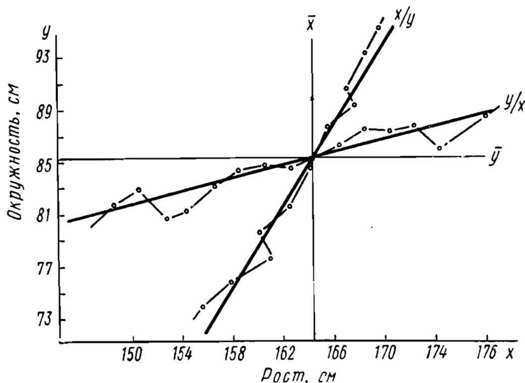
Рис. 27. Эмпирические и вычисленные по способу наименьших квадратов линии регрессии окружности груди мужчин Y по росту X и роста по окружности груди
