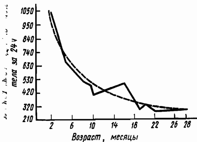
Рис. 39. Эмпирическая и вычисленная по уравнению степенной функции кривые возрастных изменений основного обмена у обезьян
