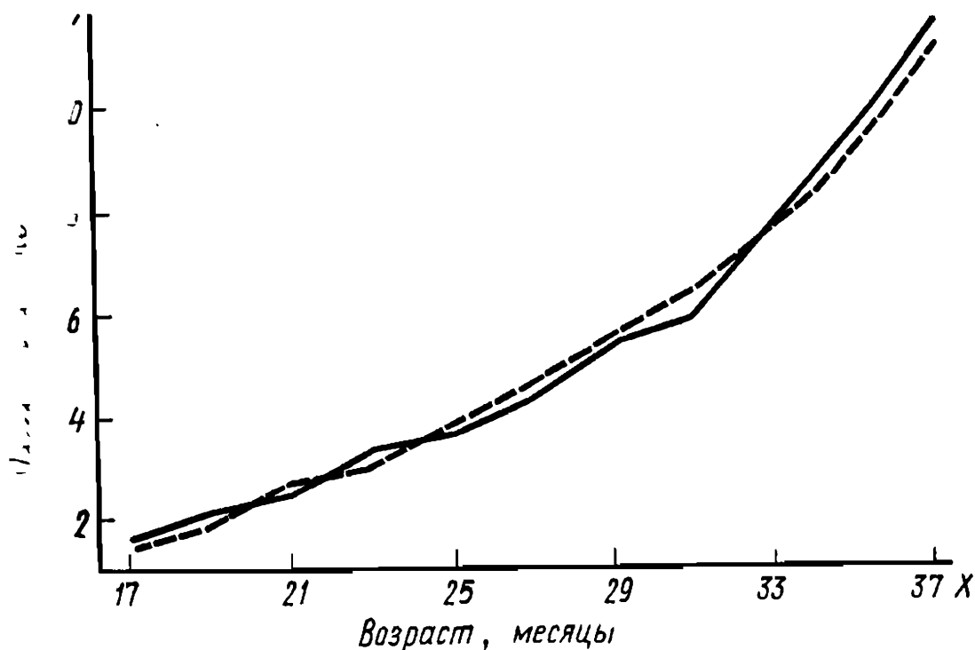
рис. 36. Эмпирическая и вычисленная по уравнению показательной функции линии регрессии возрастных изменений массы тела самцов гамадрилов в период полового созревания
