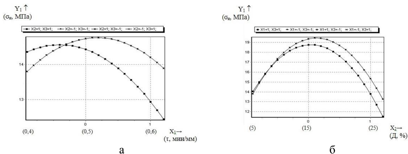
Рис. 1. Зависимости прочности плит: а - от удельной продолжительности прессования; б - от доли добавки алюмохромфосфата
