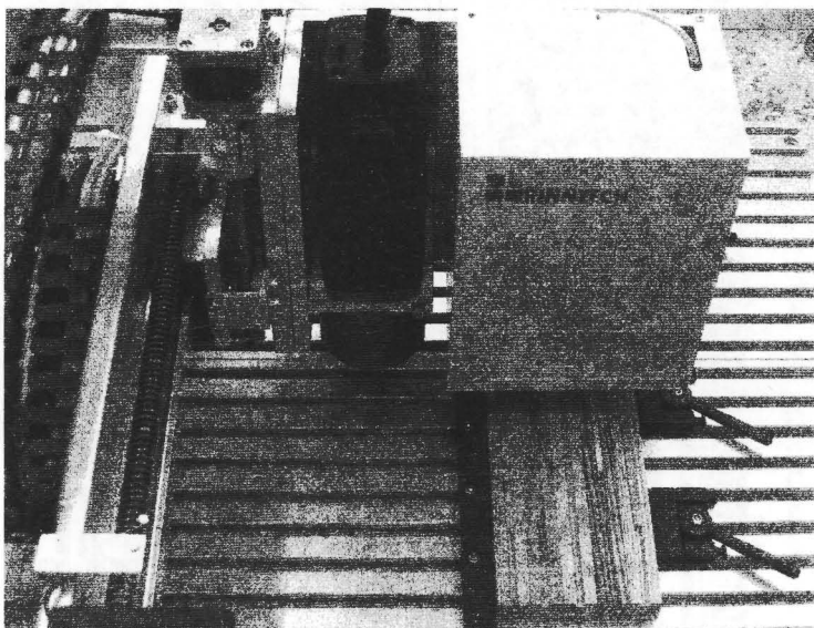
Рис. П6 Установка LIGNOSTATION позволяет получать наиболее подробную информацию о параметрах изменчивости годичных колец
