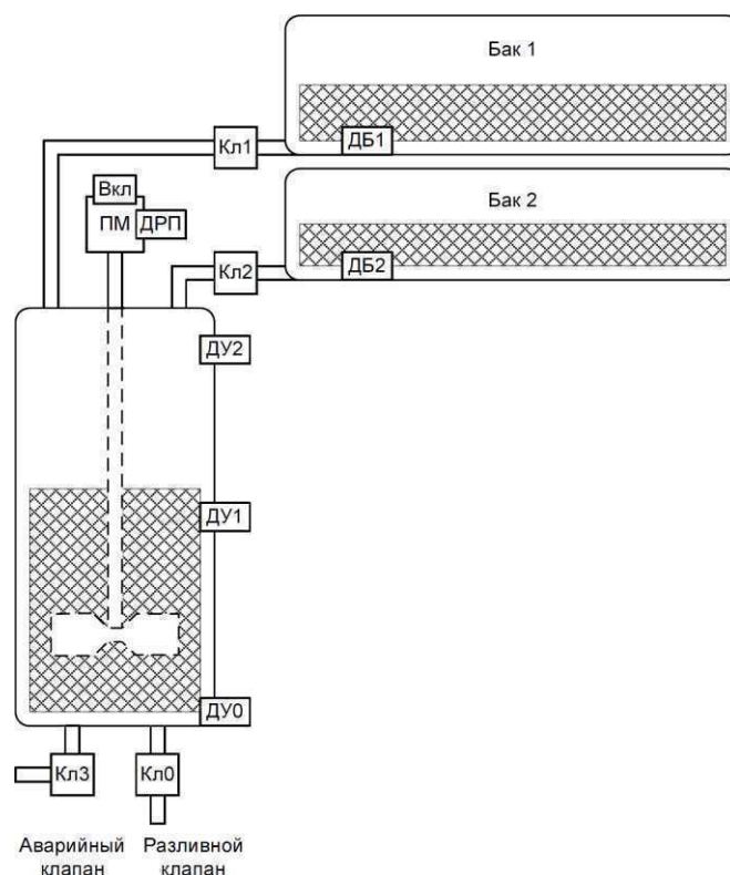
Рисунок 1 — Схематичное представление структуры установки для приготовления смесей
