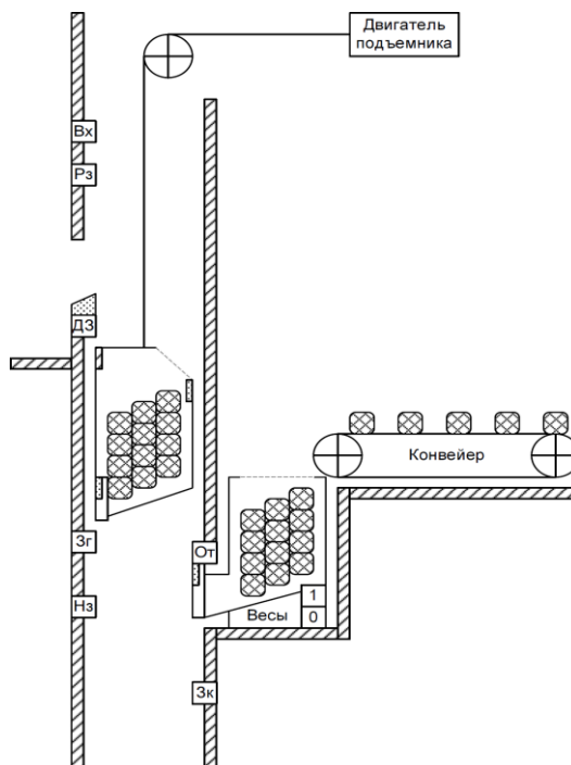
Рисунок 3 — Схематичное представление структуры шахтной скиповой подъёмной установки
