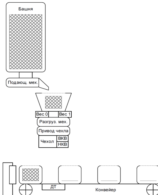
Рисунок 2 — Схематичное представление структуры установки для дозирования извести
